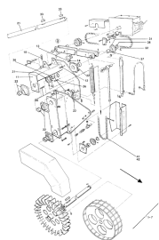
ETB-007443, Napęd od koła jezdniego (1/3)
