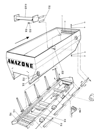
ETB-007349, Rama i skrzynia (B)
