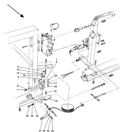
ETB-007419, Łożyskowanie do wysięgnika (3/3)
