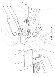
ETB-007432, Osłona przeciwbryzgowa do przedniego ślimaka rozsiewającego FS12
