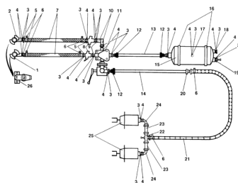
ETB-007375, Dwuobwodowy pneumatyczny układ hamulcowy (1/4)
