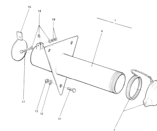
ETB-007442, Króciec wdmuchujący
