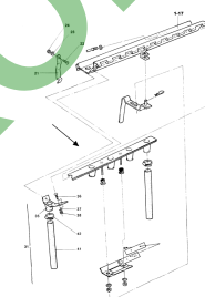
ETB-007413, Korytka rozsiewające
