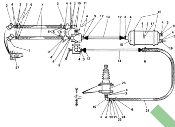
ETB-007376, Dwuobwodowy pneumatyczny układ hamulcowy (2/4)
