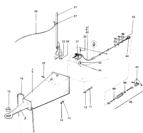
ETB-007372, Dyszel pociągowy ZG-B z hamulcem pneumatycznym
