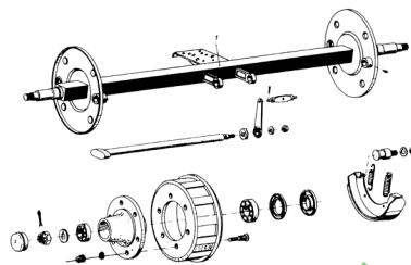
ETB-007384, Oś hamowana ZAPP STA 8X
