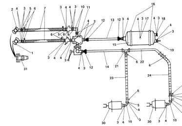
ETB-007378, Dwuobwodowy pneumatyczny układ hamulcowy (4/4)
