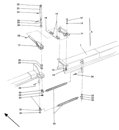
ETB-007408, Wysięgnik prawy, bez ślimaka i bez korytka
