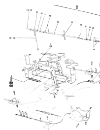
ETB-007381, Hydrauliczne elementy montażowe
