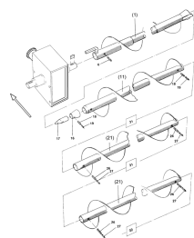
ETB-007423, Ślimaki do przedniego ślimaka rozsiewającego 12 m
