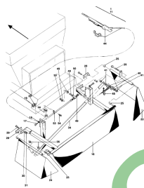
ETB-007436, Wyposażenie do zimowego utrzymania dróg i posypywarek
