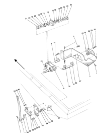
ETB-007366, Widelec sterujący do napędu rewersyjnego
