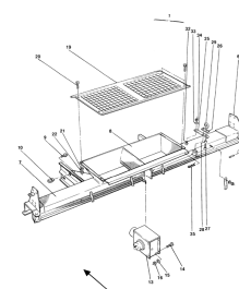
ETB-007405, Rama nośna
