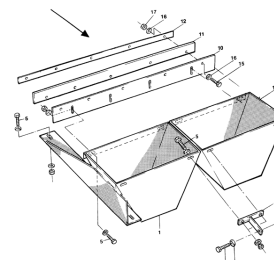
ETB-007429, Lejki
