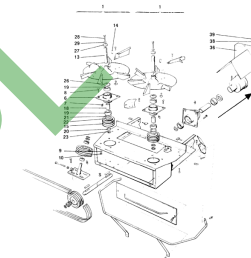
ETB-007398, Kołnierz talerzowy kompl., mechanizm rozśiewający ZG-B
