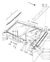
ETB-007355, Taśma
