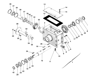
ETB-007406, Przekładnia ślimaka rozśiewającego (wszystkie typy)
