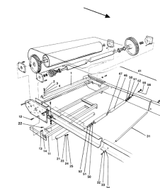
ETB-007358, Skrobak do bębna napędowego/bębna napinającego
