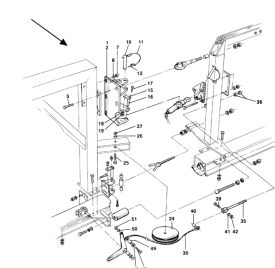
ETB-007418, Łożyszkowanie do wysięgnika (2/3)
