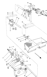
ETB-007364, Wałek napędu głównego (3/3)
