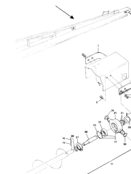
ETB-007422, Łożyskowanie ślimaka zewnętrzne, ślimak rozsiewający 12 m/łożysko wahliwe
