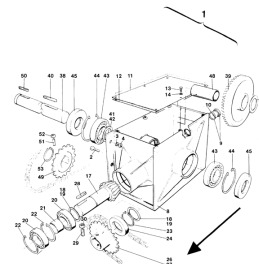
ETB-007361, Przekładnia kątowna (wszystkie typy)
