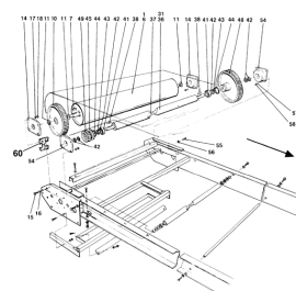
ETB-007357, Bęben napędowy, bęben napinający
