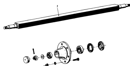
ETB-007391, Oś toczna PEITZ PL 7008
