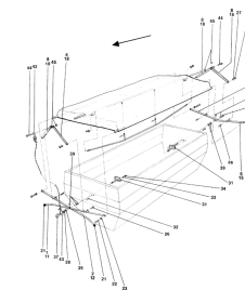
ETB-007438, Składana płandeka (2/2)
