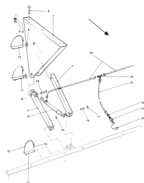
ETB-007435, Hydr. regulacja wysokości do ślimaka rozsiewającego S 200/3
