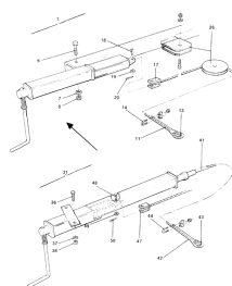
ETB-007373, Hamulec postojowy od rocznika model. 1990 tylko do osi pojedynczych
