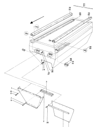
ETB-007352, Elementy montażowe na skrzyni
