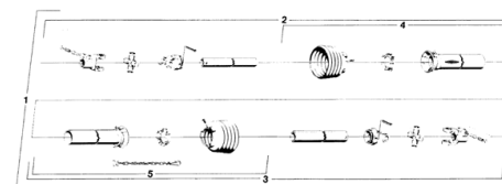
ETB-007393, Wałek przekątnikowy W 2300-SC15-1010
