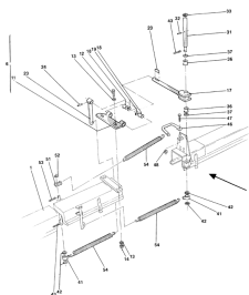
ETB-007407, Wysięgnik lewy, bez ślimaka i bez korytka
