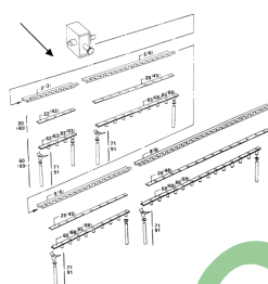
ETB-007424, Korytka rozsiewające i zasuwę do przedniego ślimaka rozsiewającego 12 m
