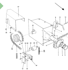
ETB-007446, Sprzęgło do napędu od koła jezdniego
