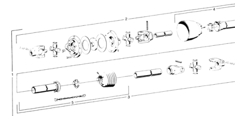
ETB-007394, Wałek przekątnikowy WVE 2370-SC15-1010
