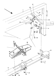
ETB-007415, Przedni ślimak rozsiewający FS12 o szerokości roboczej 12 m ZG-B 10000R
