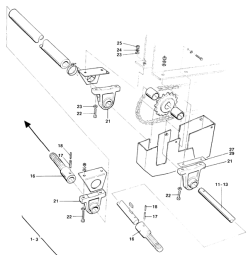
ETB-007359, Wałek napędu głównego (1/3)
