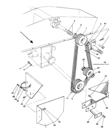
ETB-007430, Napęd pasowy do
