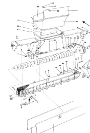
ETB-007434, Ślimak rozsiewający S 200/3 (2/2)
