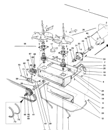
ETB-007397, Dwutarczowy mechanizm rozśiewający
