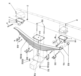
ETB-007382, Zawieszenie (1/2)
