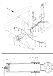
ETB-007420, Siłownik hydrauliczny do składania wysięgników
