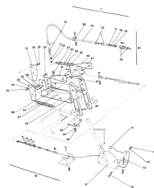
ETB-007379, Hydrauliczny układ hamulcowy (1/2)
