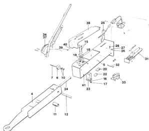
ETB-007371, Dyszel pociągowy z urządzeniem najazdowym AER H 80
