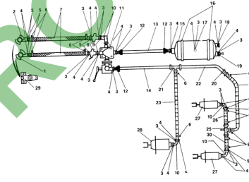
ETB-007377, Dwuobwodowy pneumatyczny układ hamulcowy (3/4)
