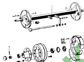
ETB-007385, Oś hamowana PEITZ ERA-KV 8008 (1/2)
