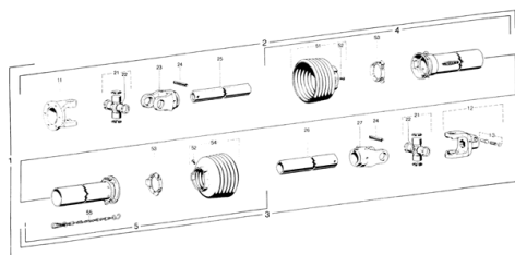
ETB-007363, Wałek przekaźnikowy
