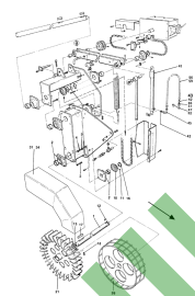
ETB-007445, Napęd od koła jezdniego (3/3)
