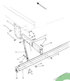
ETB-007448, Zabezpieczenie przeciwwjazdowe
