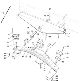
ETB-007383, Zawieszenie (2/2)
