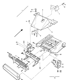
ETB-007351, Blacha kierująca
