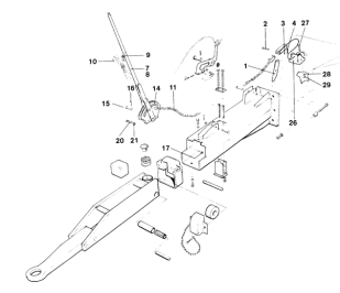
ETB-007370, Dyszel pociągowy z urządzeniem najazdowym AVE H 80 (2/2)
