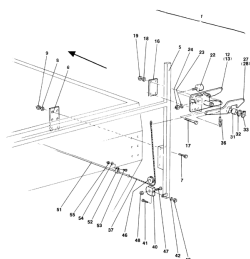
ETB-007431, Urządzenie transportowe do przedniego ślimaka rozsiewającego FS12
