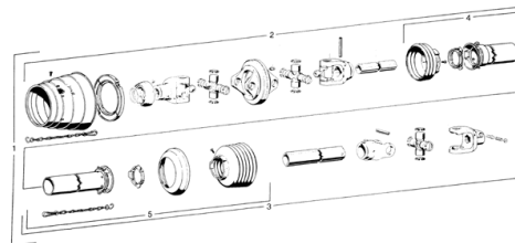
ETB-007396, Wałek przekątnikowy WWE 2380-SD15-1010
