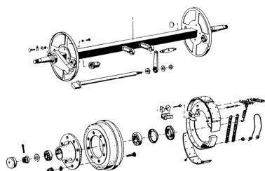
ETB-007387, Oś hamowana PEITZ ERA 7008 (1/2)
