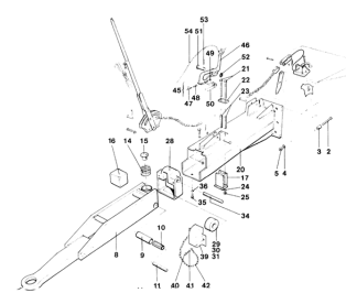
ETB-007369, Dyszel pociągowy z urządzeniem najazdowym AVE H 80 (1/2)
