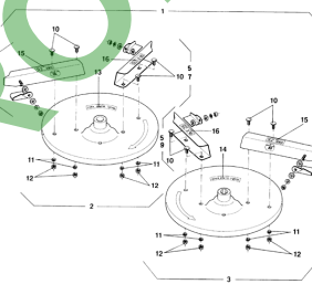
ETB-007401, Specjalna tarcza rozśiewająca S3
