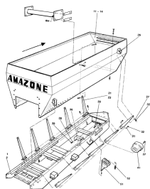
ETB-007347, Rama i skrzynia (A)
