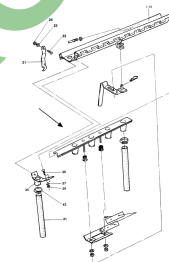
ETB-007425, Elementy montażowe do korytek rozsiewających
