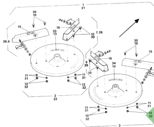
ETB-007400, Specjalna tarcza rozśiewająca S2 / S2E
