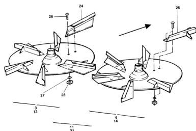
ETB-007399, Tarcze rozśiewające ZG-B
