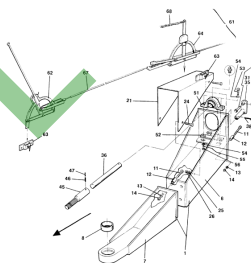
ETB-007374, Wygięty dyszel pociągowy (tylko na rynek francuski i belgijski)
