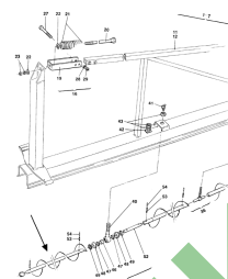
ETB-007421, Wysięgnik kompl./łożyskowanie ślimaka środkowe
