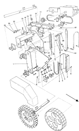
ETB-007444, Napęd od koła jezdniego (2/3)
