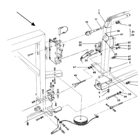
ETB-007417, Łożyszkowanie do wysięgnika (1/3)
