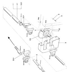
ETB-007360, Wałek napędu głównego (2/3)
