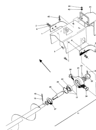
ETB-007409, Łożyszkowanie wysięgnika końcowego/łożysko wahliwe
