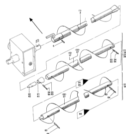
ETB-007411, Ślimak rozsiewający do ślimaków rozsiewających o szerokości roboczej 6 m i 8 m
