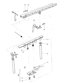
ETB-007414, Zasuw węży
