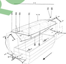
ETB-007437, Składana płandeka (1/2)
